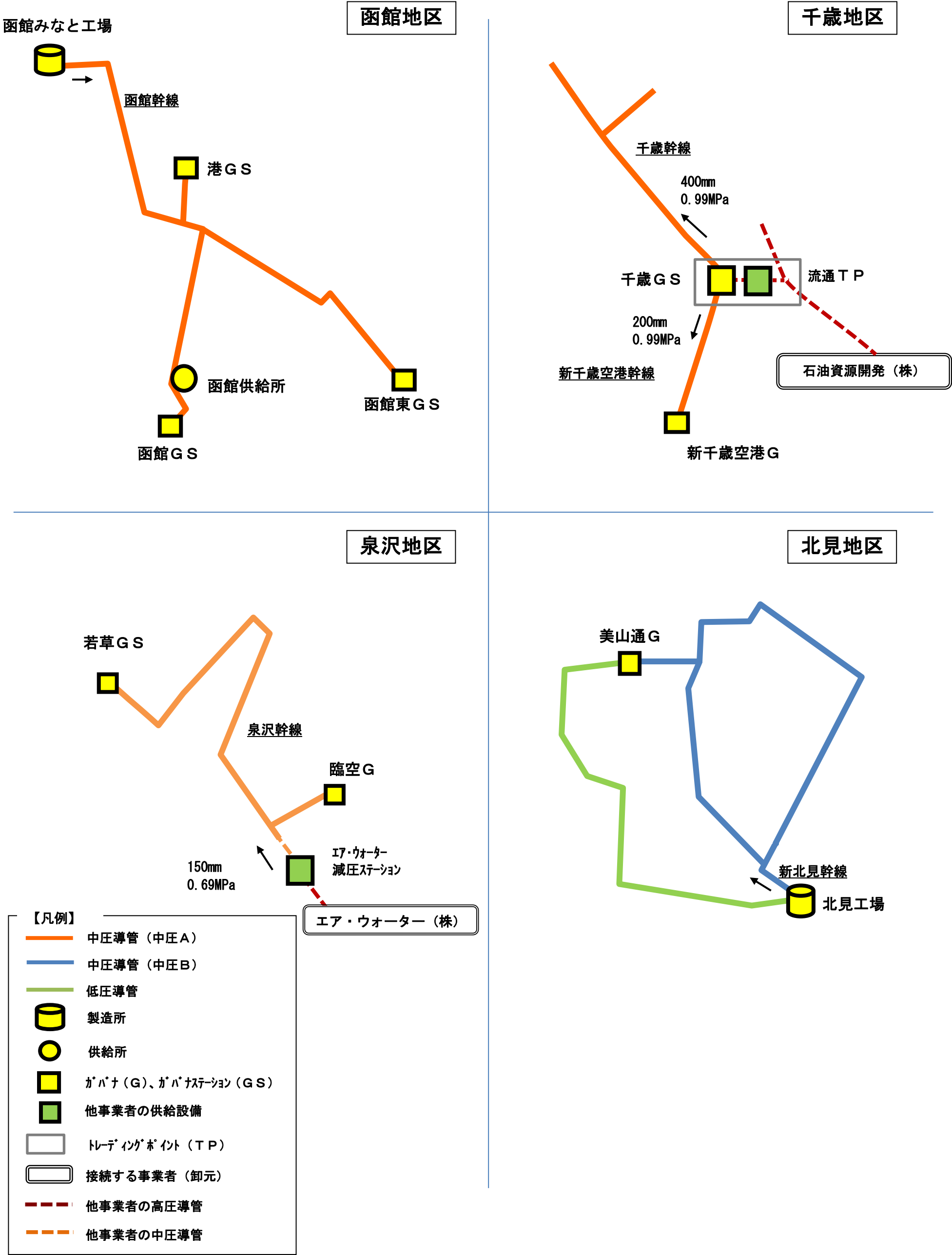
(一般ガス導管事業) 第8表 主要導管図
