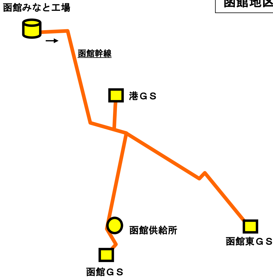
(一般ガス導管事業) 第8表 主要導管図
