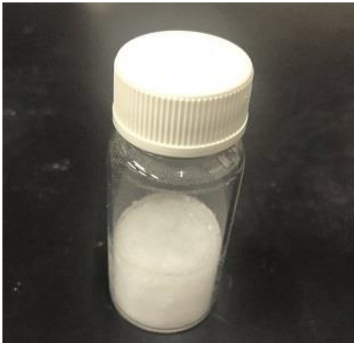
結晶化したクラスレート水ドレート
